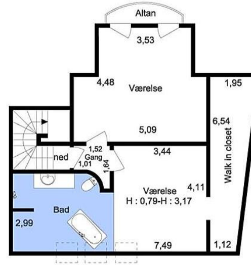
1. sal
