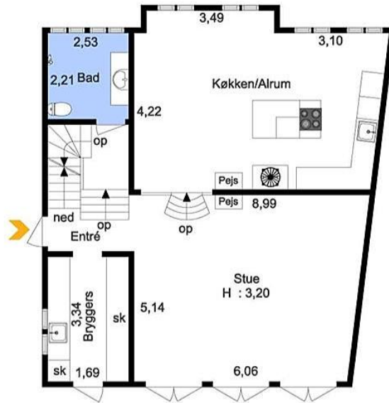
Stueplan
