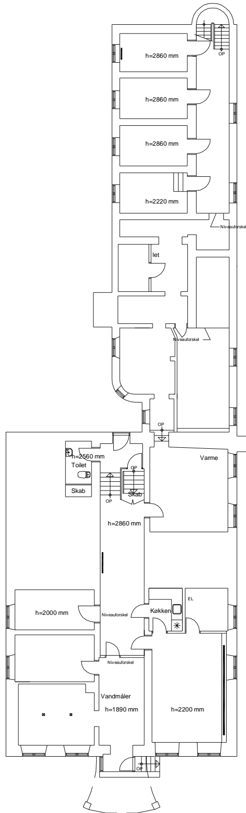
Rudkøbing gamle rådhus - kælderplan
